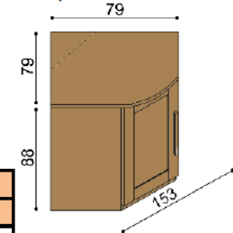
Komoda PAVLA C1SL (P) - dvířka prosklená, sklo čiré, 3 police
